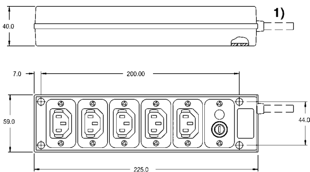
Stripbloc 4740.3X00
