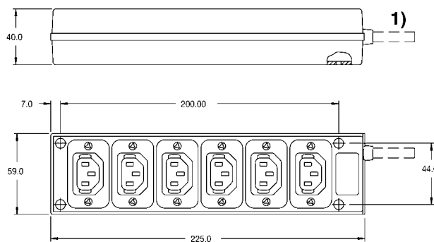
Stripbloc 4740.4X00
